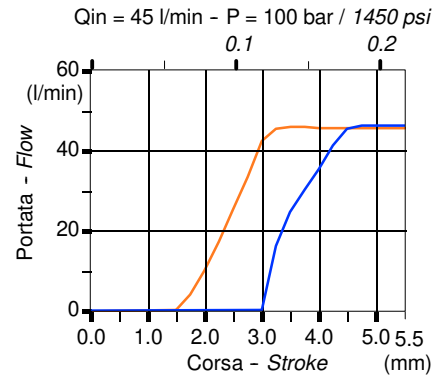
Sensibilità cursore 1 - Spool 1 metering
